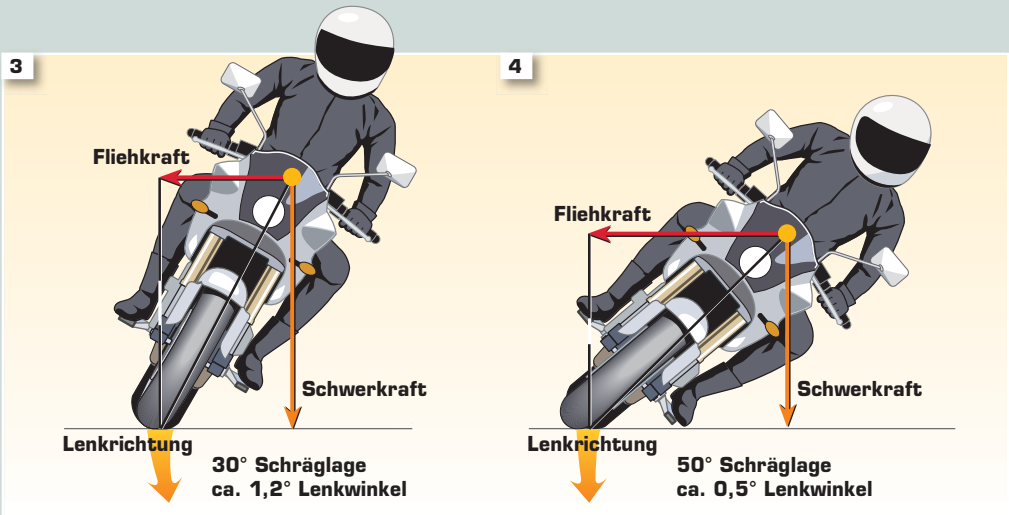
Grafik 3: Mit 30 Grad Schräglage ist man bei trockener Straße auf der sicheren Seite. Zu sehen daran, dass die Fliehkraft (roter Pfeil) noch deutlich kleiner ist als die Schwerkraft (gelber Pfeil). Gut zu erkennen: der Refenaufstandspunkt wandert mit steigender Schräglage nach außen.
