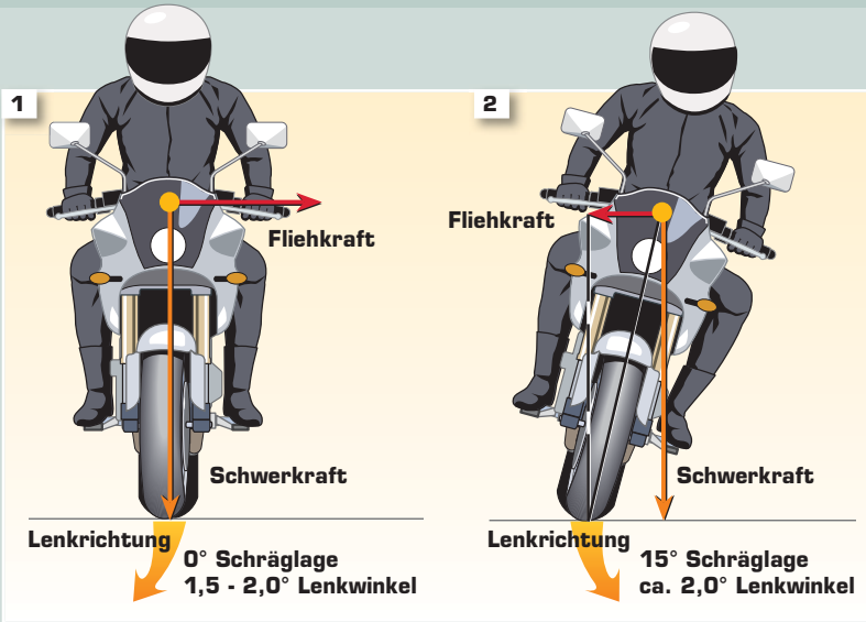
Grafik 1: Meist unbewusst erfolgt der Lenkimpuls vor einer Linkskurve zunächst nach rechts, worauf die Fliehkraft den Schwerpunkt aus Motorrad und Fahrer nach links kippt. Je größer der Lenkimpuls/Lenkwinkel ausfällt, desto abrupter klappt die Maschine in Schräglage, was sich auf einer verkehrsfreien, übersichtlichen Strecke ausprobieren lässt.
